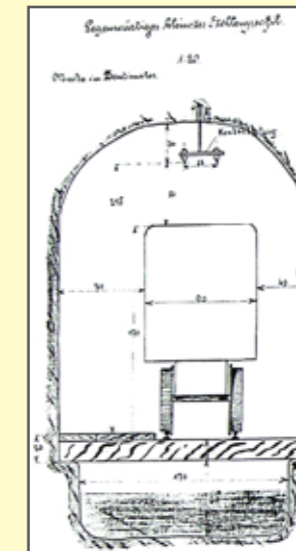
Schema originale della sezione della galleria.
