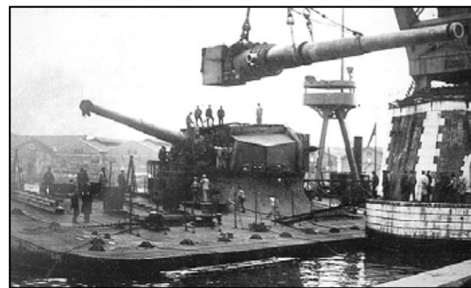
Pontone armato Faà di Bruno
