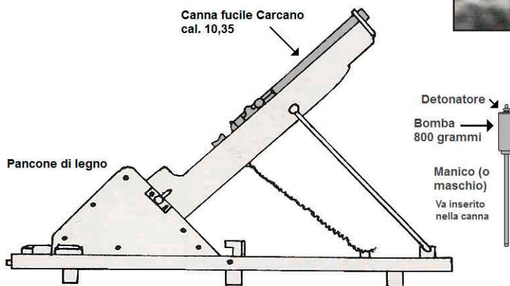
Lanciabombe Carcano 1969 cal. 10,35
