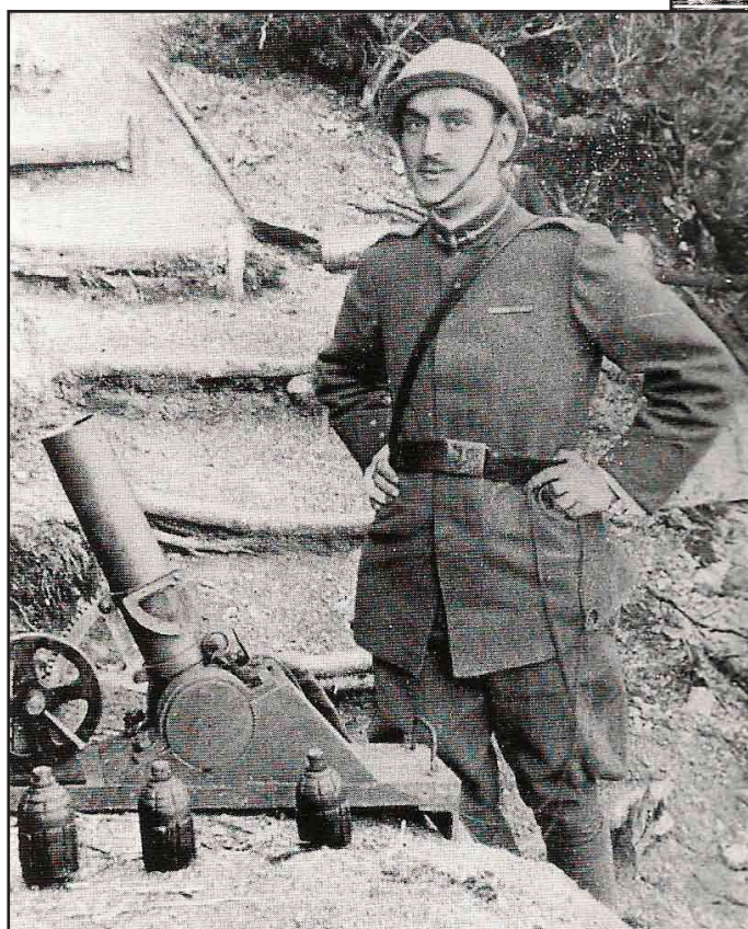
Lanciabombe Torretta cal. 65
